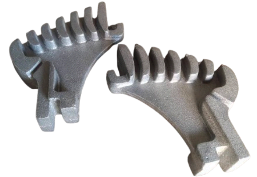
NAME : GRATE BAR MATERIAL : 1.4777
