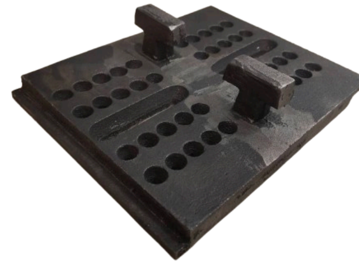
NAME : GRATE BAR MATERIAL : FCD450
